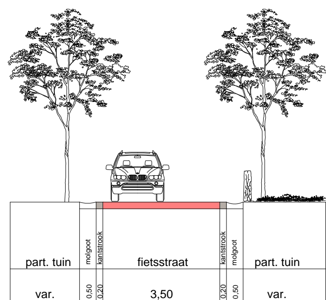
Wooldrikshoekweg (Lammertsweg - Heutinkhoekweg) nieuw dwarsprofiel (A - A)
