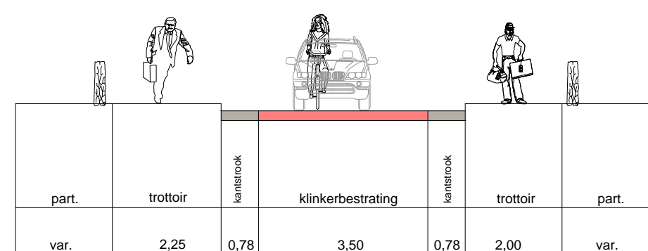
Tegelerweg (Rechterlaan - Heutinkstraat) nieuw dwarsprofiel (H - H)
