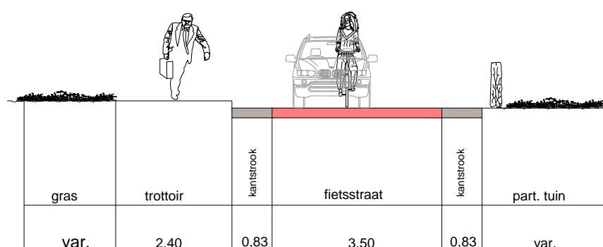
Tegelerweg (wooldrikshoekweg - van der Waalslaan) nieuw dwarsprofiel (D - D)
