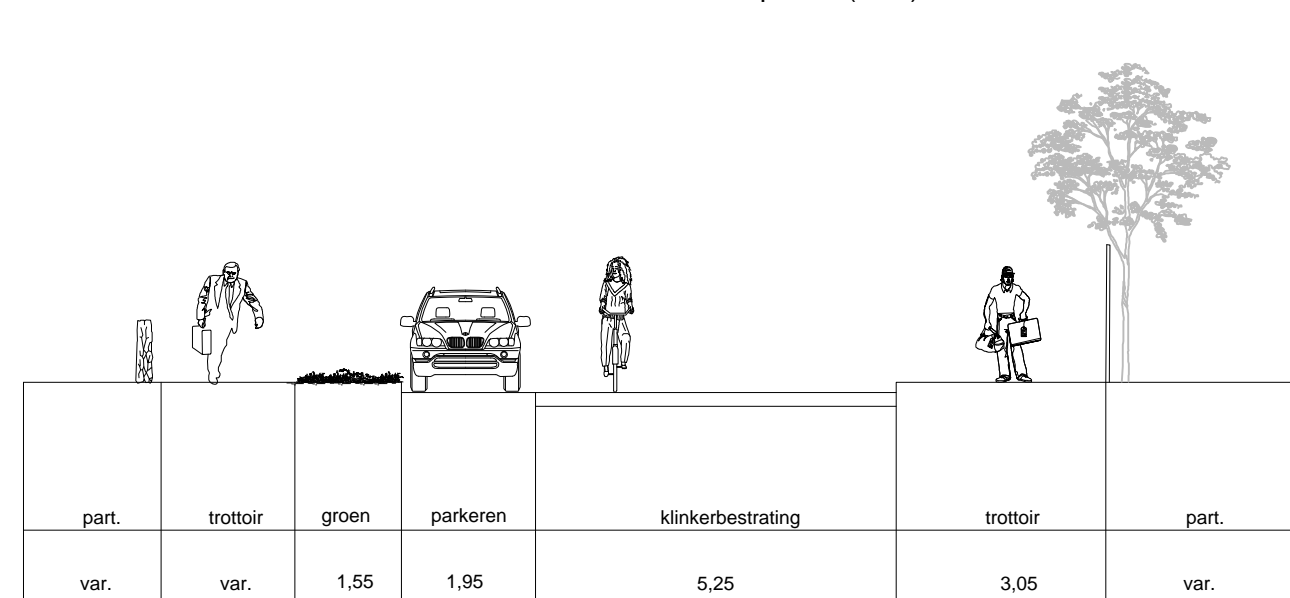
Heutinkstraat (Tegelerweg - Hogelandsingel) bestaand dwarsprofiel (K - K)
