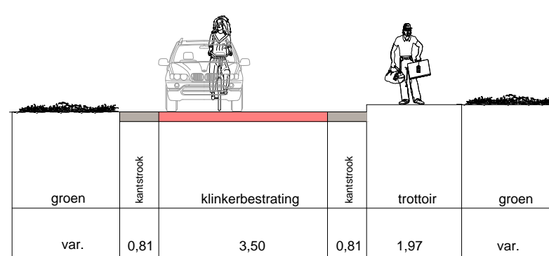
Tegelerweg (Lorentzlaan - Rechterlaan) nieuw dwarsprofiel (G - G)
