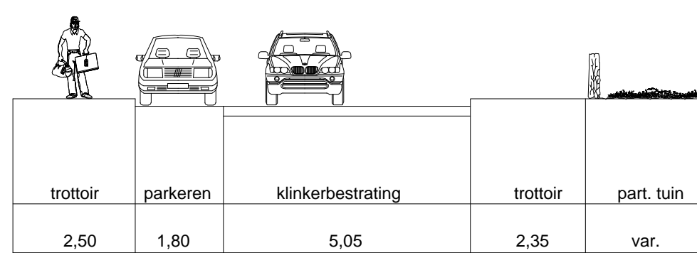
Wooldrikshoekweg (Tegelerweg - Lammertsweg) bestaand dwarsprofiel (B - B)
