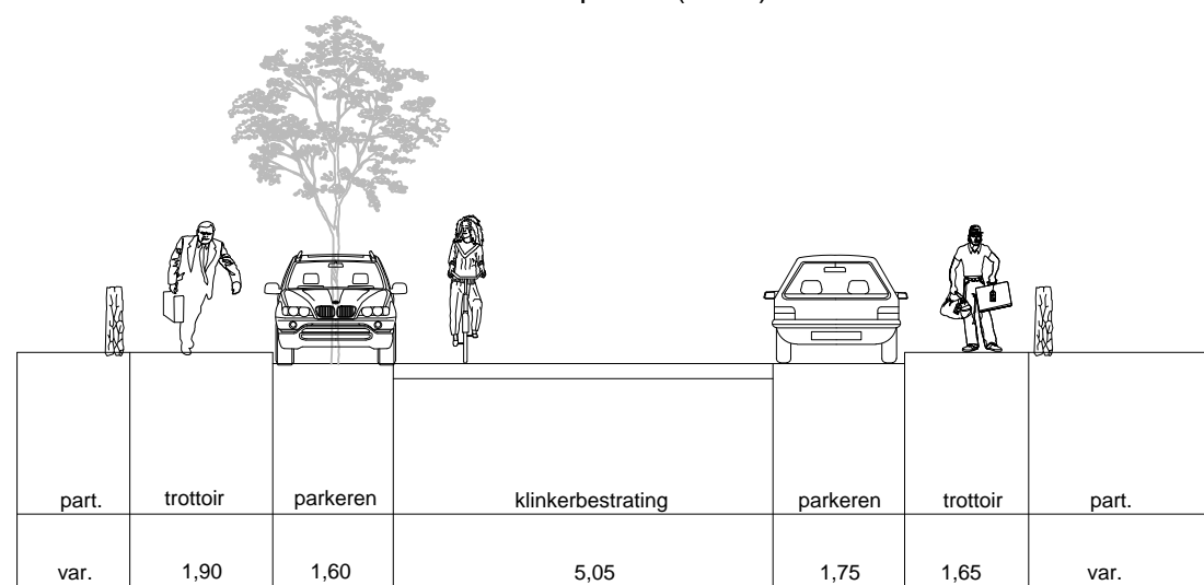
Heutinkstraat (Tegelerweg - Hogelandsingel) bestaand dwarsprofiel (J - J)
