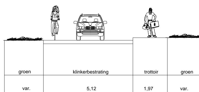
Tegelerweg (Lorentzlaan - Rechterlaan) bestaand dwarsprofiel (G - G)
