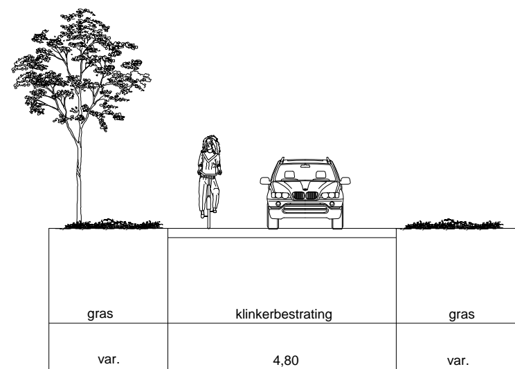
Tegelerweg (van der Waalslaan - Van 't Hofflaan) bestaand dwarsprofiel (E - E)
