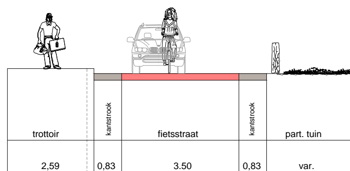
Tegelerweg (wooldrikshoekweg - van der Waalslaan) nieuw dwarsprofiel (C - C)
