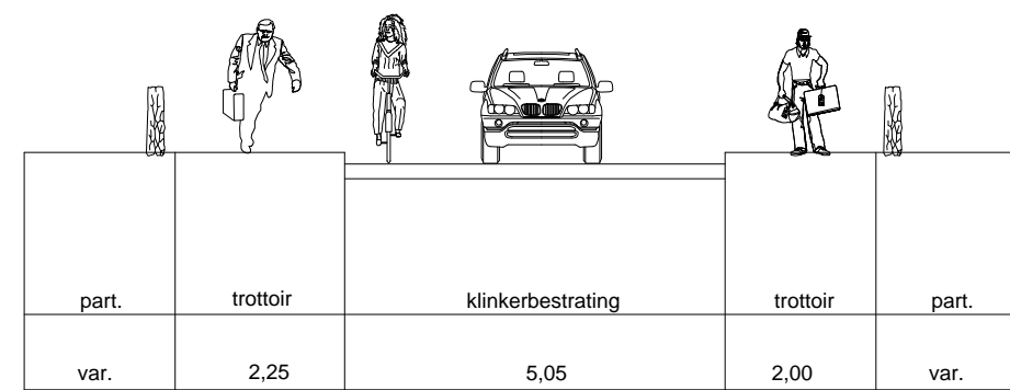
Tegelerweg (Rechterlaan - Heutinkstraat) bestaand dwarsprofiel (H - H)
