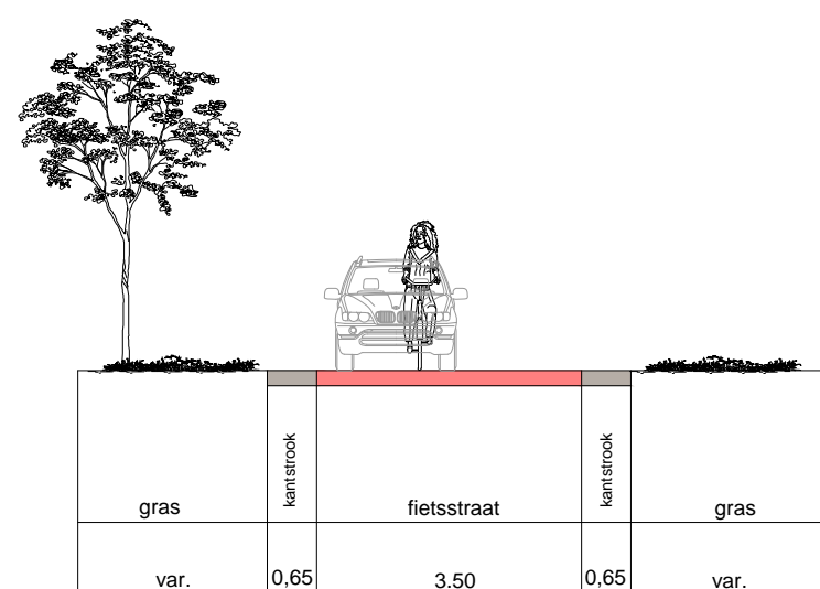
Tegelerweg (van der Waalslaan - Van 't Hofflaan) nieuw dwarsprofiel (E - E)
