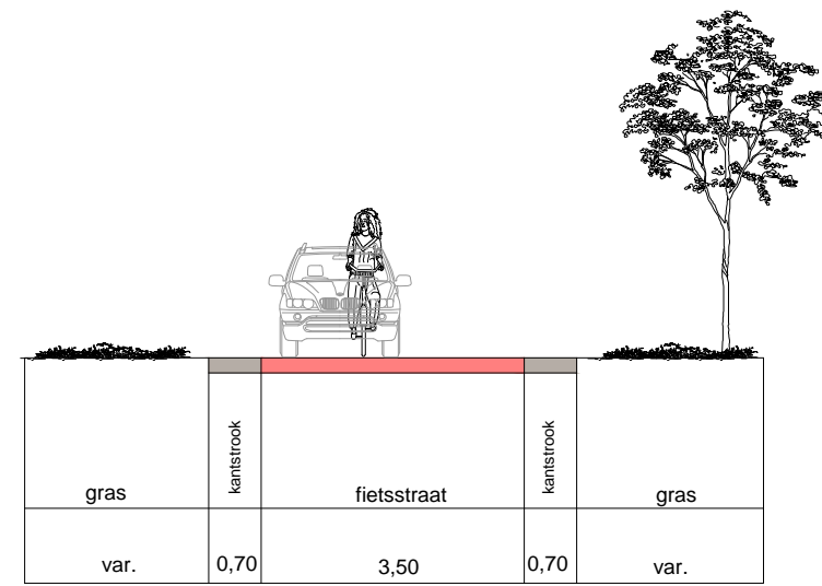
Tegelerweg (Van 't Hofflaan - Lorentzlaan) nieuw dwarsprofiel (F - F)
