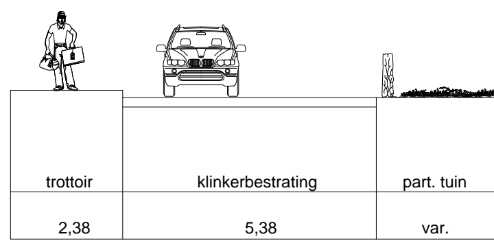
Tegelerweg (wooldrikshoekweg - van der Waalslaan) bestaand dwarsprofiel (C - C)
