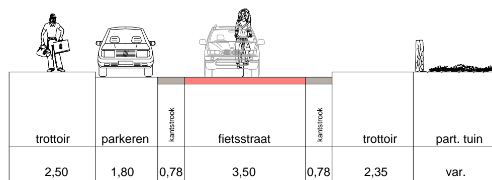
Wooldrikshoekweg (Tegelerweg - Lammertsweg) nieuw dwarsprofiel (B - B)
