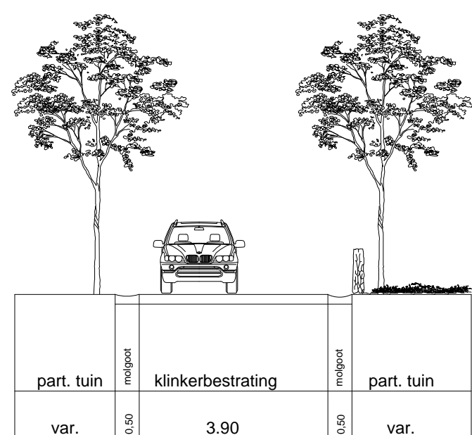
Wooldrikshoekweg (Lammertsweg - Heutinkhoekweg) bestaand dwarsprofiel (A - A)
