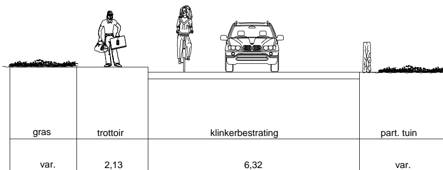
Tegelerweg (wooldrikshoekweg - van der Waalslaan) bestaand dwarsprofiel (D - D)
