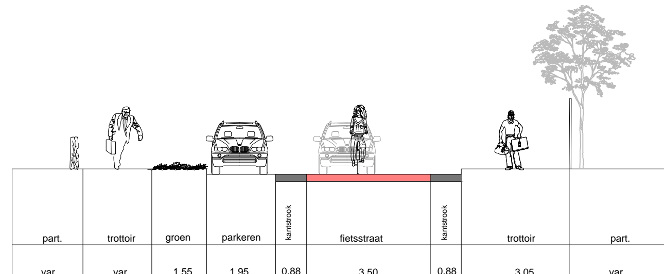
Heutinkstraat (Tegelerweg - Hogelandsingel) nieuw dwarsprofiel (K - K)
