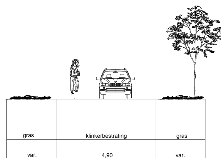
Tegelerweg (Van 't Hofflaan - Lorentzlaan) bestaand dwarsprofiel (F - F)
