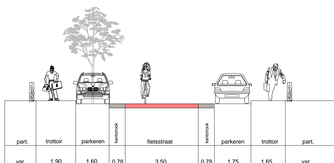
Heutinkstraat (Tegelerweg - Hogelandsingel) nieuw dwarsprofiel (J - J)
